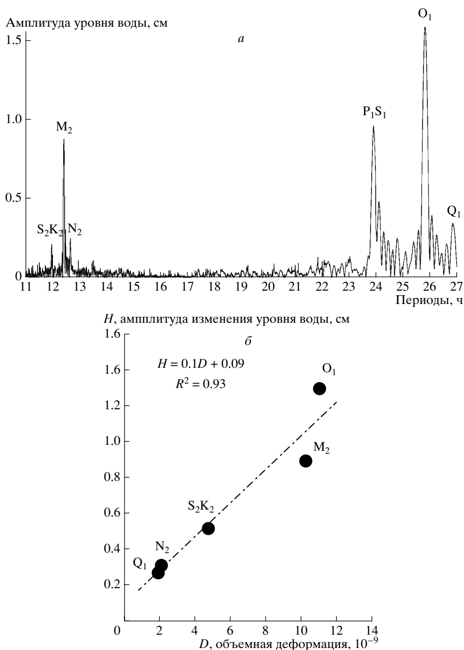
Рис. 3. Характеристика приливного отклика уровня воды в скважине ЮЗ-5: a – периодограмма вариаций уровня воды в приливном диапазоне 11–27 ч; b – зависимость выделенных приливных амплитуд в изменениях уровня воды от величин теоретической приливной деформации (табл. 2).
