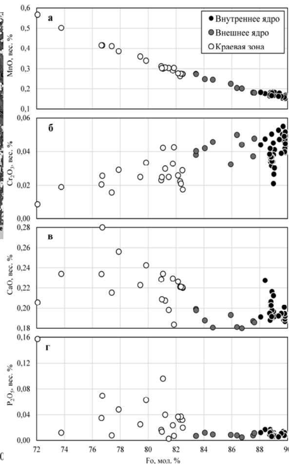
Рис. 2. Зависимость концентрации микроэлементов от содержания форстерита в оливинах из высоко-Mg высоко-K базальта побочного извержения 1941 года на вулкане Толбачик. Черные кружки – внутреннее ядро кристалла, серые кружки – внешнее ядро, и белые кружки – краевая зона.
