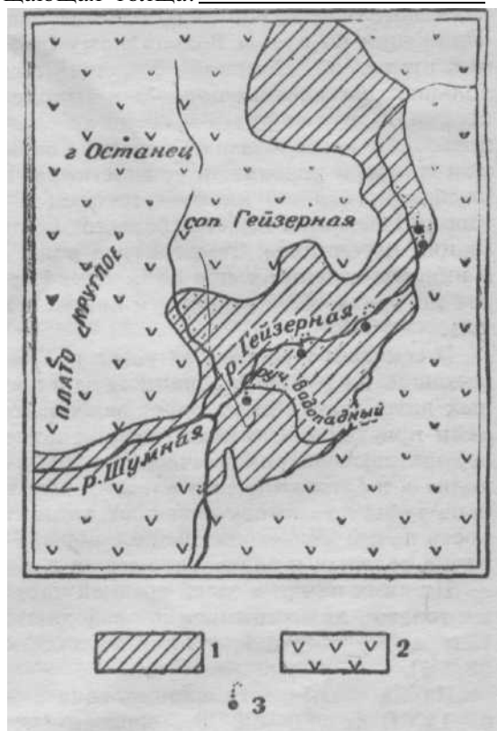
Схематическая геологическая карта района Долины Гейзеров.
