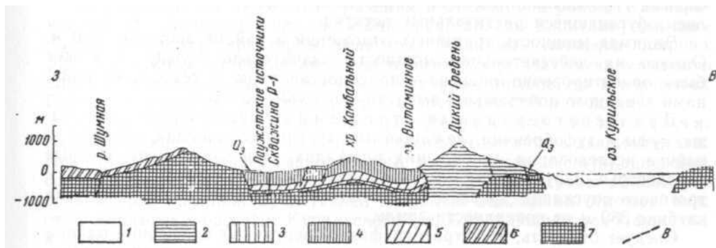
Рис. 1. Схематический геологический разрез через район Паужетских источников на Южной Камчатке. Составил В. В. Аверьев по данным маршрутных исследований 1957—1958 гг. и материалам предыдущих работ.
