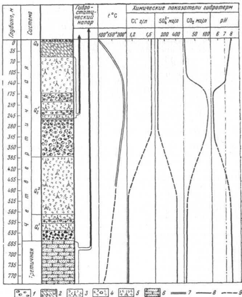
Рис. 3. Сводная характеристика скважины Р-1 на Паужетских источниках.
