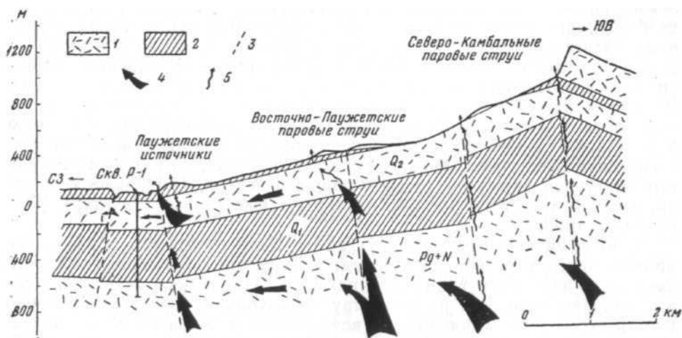
Рис. 2. Схема разгрузки Паужетских гидротерм.
