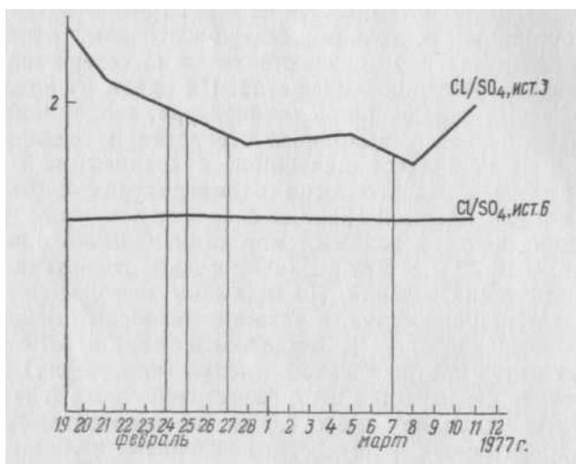
Рис. 2. Отношения Cl/SO 4 в источниках 3 и 6 и землетрясения февраля-марта 1977 г.
