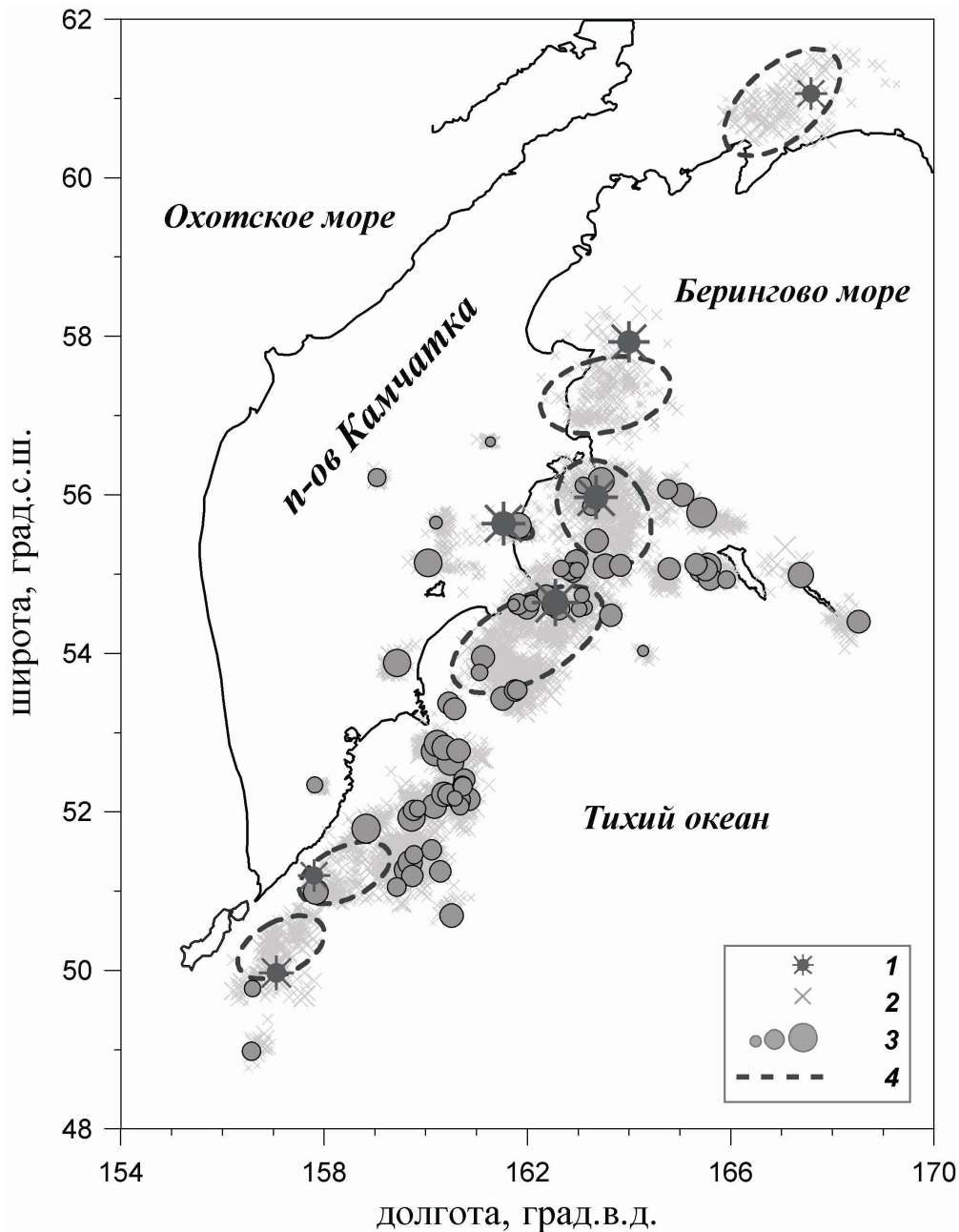
Рис. 3. Схема пространственного расположения областей афтершоковых последовательностей, эпицентров главных землетрясений и их афтершоков. 1 - эпицентр главного события с K \geq 15.0 ; 2, 3 - эпицентры афтершоков и главных событий, масштабируемых по энергетическому классу: 10.7 \leq K \leq 12.1 , 12.1 < K \leq 13.5 и 13.5 < K \leq 14.9 ; 4 - области афтершоковых последовательностей.
