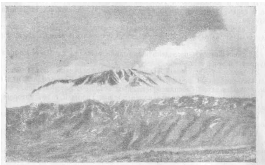
Рис. 4. Вулкан Плоский Толбачик с северо-восточной стороны. Из кратера частые взрывы-выбросы, сопровождающиеся выделениями водяных паров и газов в интервалах через 1—4 мин.
