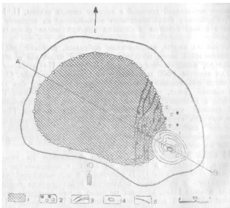
Рис. 2. План колодцеобразного провала в кратере вулкана Плоский Толбачик.
