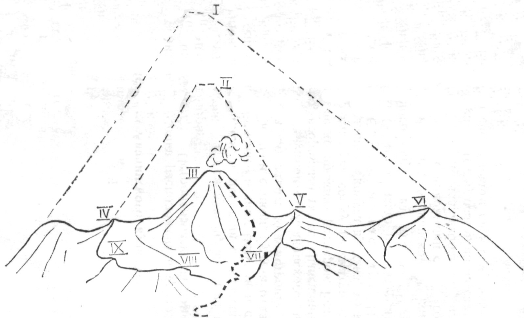
I. Первоначальный конус Авачинского вулкана. II. Вторичный конус. III. Современный конус. IV. Сарай. V. Сомма. VI Козельская сопка. VII. Скала Кутхи. VIII. С. Игорева. IX. С. Монастырь. ----- Путь экспедиции в 1923 году.
